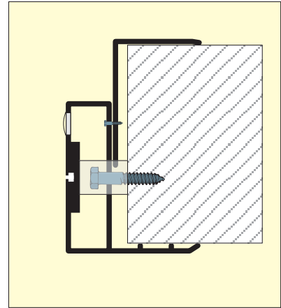
3. PK3 aluminium Foder 130-170 mm
