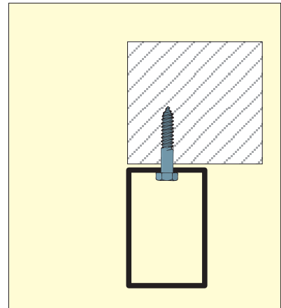
6. PK6 fyrkantskarm stål/alu 40x60 mm
