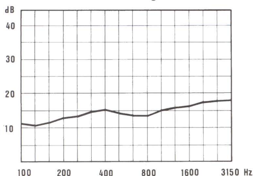
Reduktionstalsmätning PVC-remsor 400/4/200
